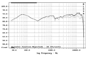
Raumakustik-Frequenzgang: Triangle
